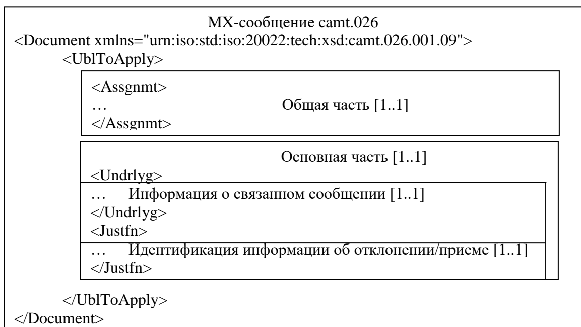
Рисунок 1 – Структура МХ-сообщения camt.026
